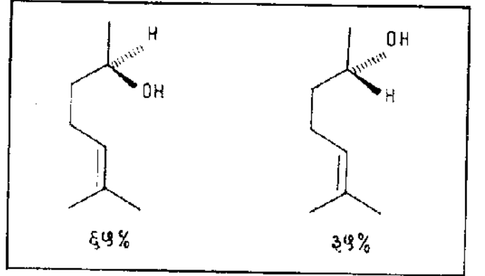
१८. दोन्ही त्रिमितीय समघटकांचे मिश्रण
